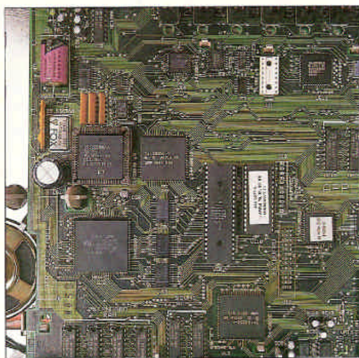
La zona più densa della piastra dell'Apple IIGS. In primo piano (al centro) il 'tradizionale' 65C816 (incompatibile 6502), a fianco (verso destra) la ROM e il controller della tastiera. Sotto il processore sonoro, a sinistra il Mega II (un Apple IIe in un chip) e più in alto il controller video e il Fast Processor Interface. Ancora più su si notano la pila al litio che mantiene l'orologio e il control panel, l'Integrated WOZ Machine (dischi), il game pad e lo slotmaker che completano la capacità di emulazione di questa macchina.
