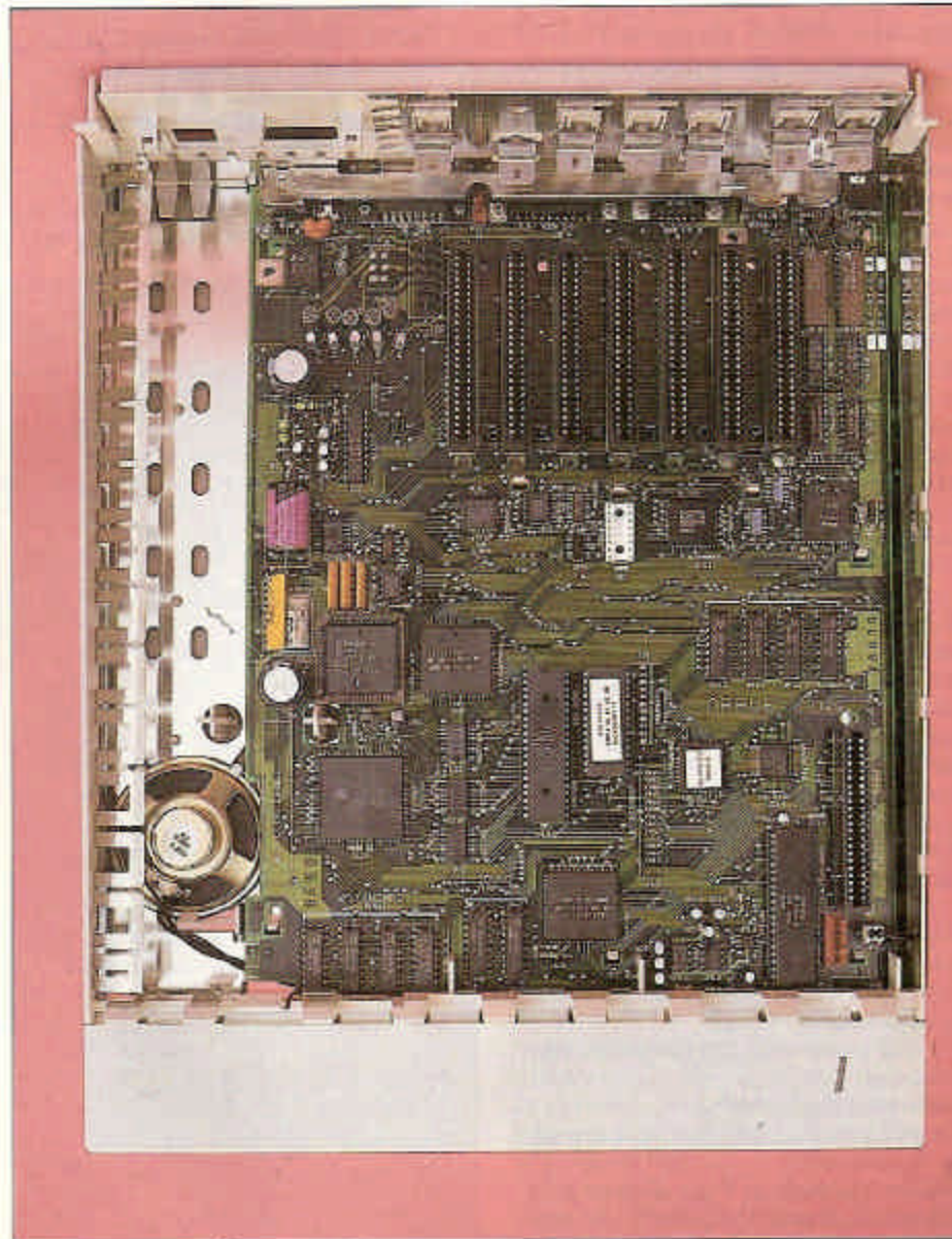
Tolto l'alimentatore, tenuto da un aggancio a scatto, si può ammirare l'eleganza della piastra madre, il filo è quello che collega l'altoparlante interno. Negli USA la piastra madre viene venduta da sola come grade dell'Apple IIe.
