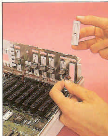
Le feritoie di uscita degli eventuali cavi o per montare i connettori standard RS 232 sono chiuse da tappi di plastica bloccati da una clip a baionetta. Se avessero realizzato pure una sede dove mettere i copercchi tolti sarebbe stato veramente il massimo.
